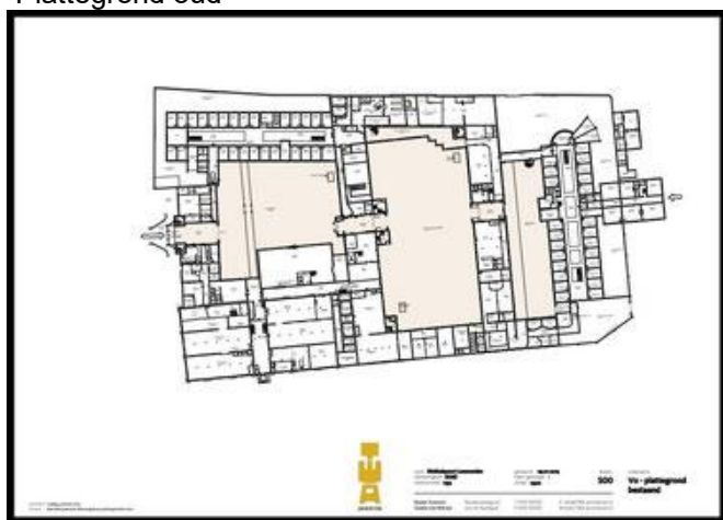
Plattegrond oud
